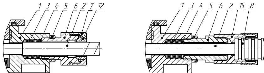
в) монтаж бронированным кабелем в кабельном вводе КВБ17
