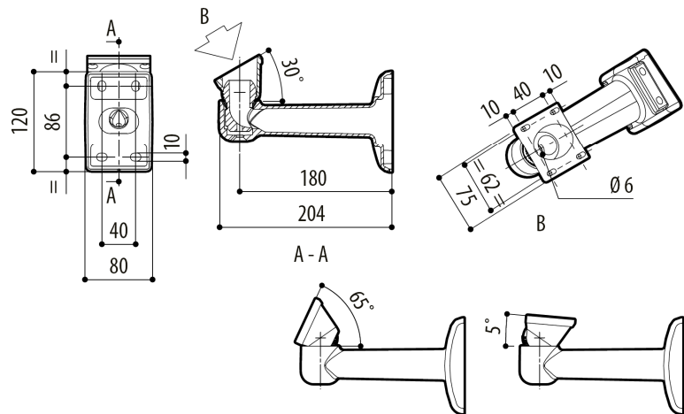
Рисунок 2. Габаритные размеры кронштейна.
